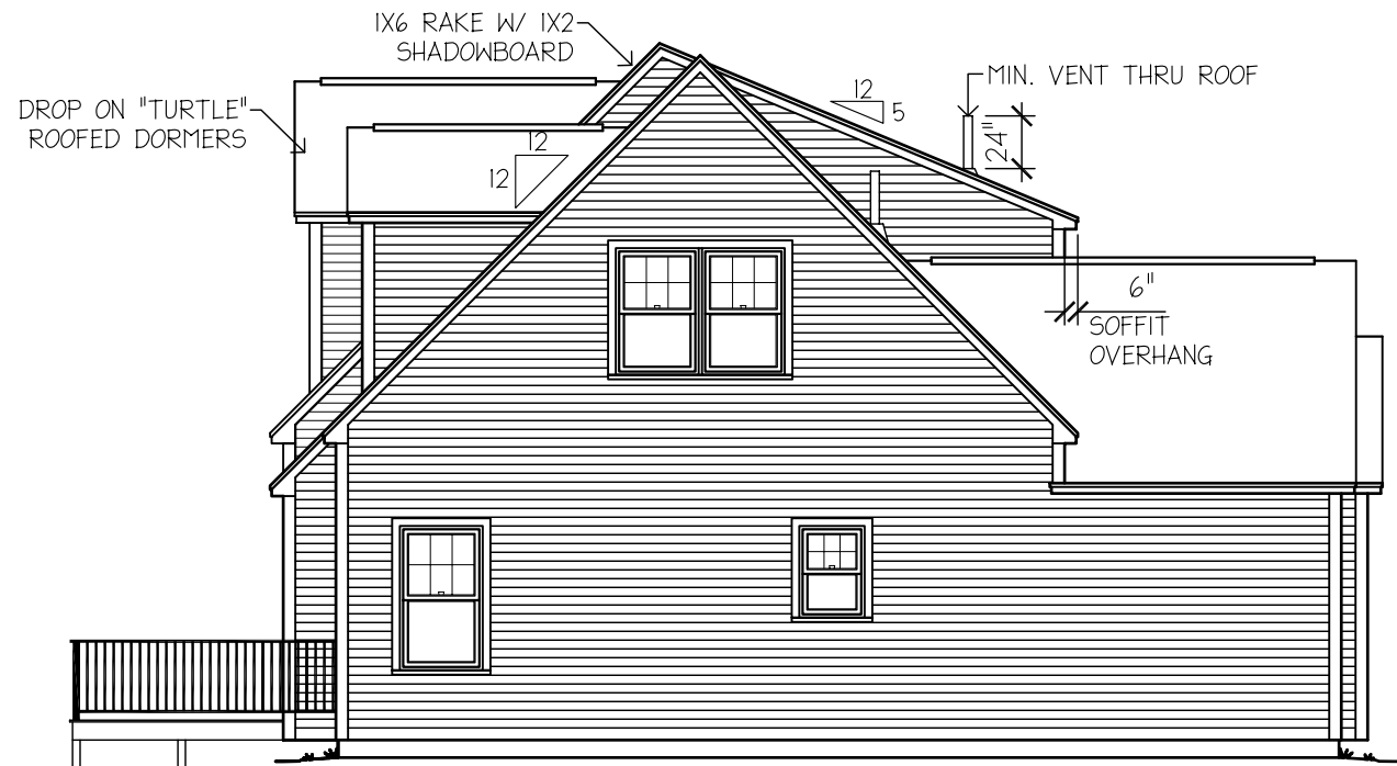
E-3 LEFT ELEVATION SCALE: 1/8" = 1'-0"
